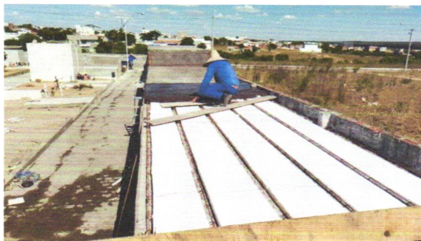
FOTO 06 - Laje pré-fabricada treliçada para piso ou cobertura, intereixo 38cm, h=12cm, el. enchimento em EPS h=8cm, inclusive escoramento em madeira e capeamento 4cm.
